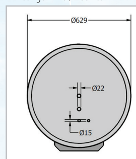
Afmetingen 120 / 200 liter
