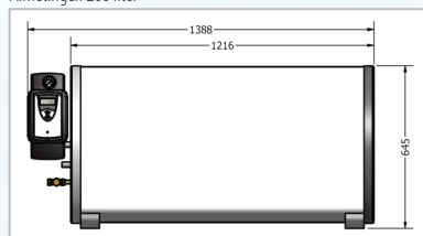
Afmetingen 200 liter
